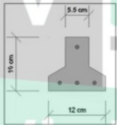
Vigueta Pretensada
